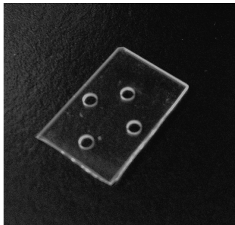
図2 0.5 mm 厚の合成石英基板に作製した微細流路中に \text{SnO}_2/\text{SiO}_2 (10 nm/10 nm) のコアシェルナノワイヤを成長させたナノワイヤデバイス
