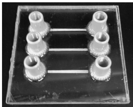
図3 ポリメタクリル酸メチル樹脂 (PMMA) に酸化亜鉛ナノワイヤを成長させたナノワイヤデバイス
