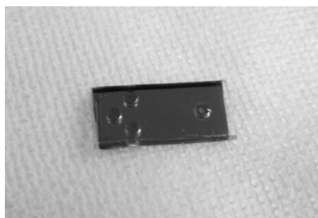
図1 Si基板上のSnO 2 ナノワイヤとポリジメチルシロキサン（PDMS）微細流路を組み合わせたナノワイヤデバイス
