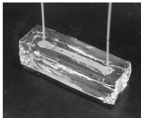
図4 PDMS に埋め込んだナノワイヤと、ヘリンボーン構造を持つ微細流路を作製した PDMS を貼り合わせたナノワイヤデバイス
