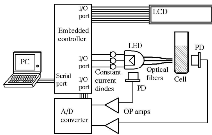
図: 装置のブロック図
